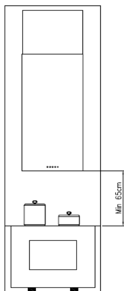
RUBIK ISOLA 40 (27kg)
